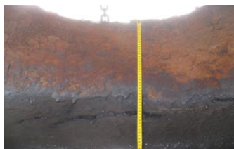
CENTRO VOLTA ALFABLOCK® DOPO 3 SETTIMANE DI USURA (foto 3)
