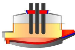
FOUR À ARC ÉLECTRIQUE
